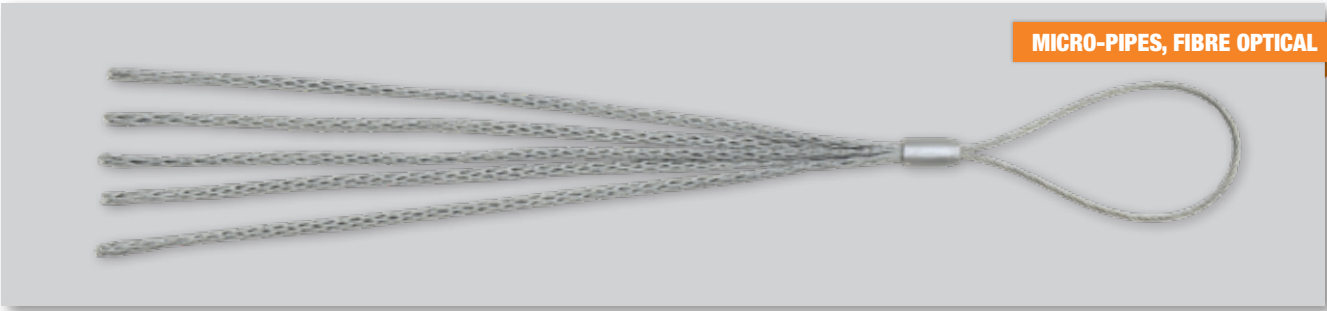
[EN] Pulling grip with single eye, for 5 micro-pipes of fibre optical cables [D] Fünffach-Kabelziehstrumpf mit einer Zugöse für 5 Mikro-Rohre für Lichtwellenleiter [E] Malla de tiro con un lazo, para 5 micro-tubos de cables de fibra óptica [F] Chaussette de tirage avec simple boucle, pour les 5 micro-tubes de câbles de fibre optique [I] Calza di tiro con un'asola, per 5 micro-tubi di cavi a fibre ottiche
